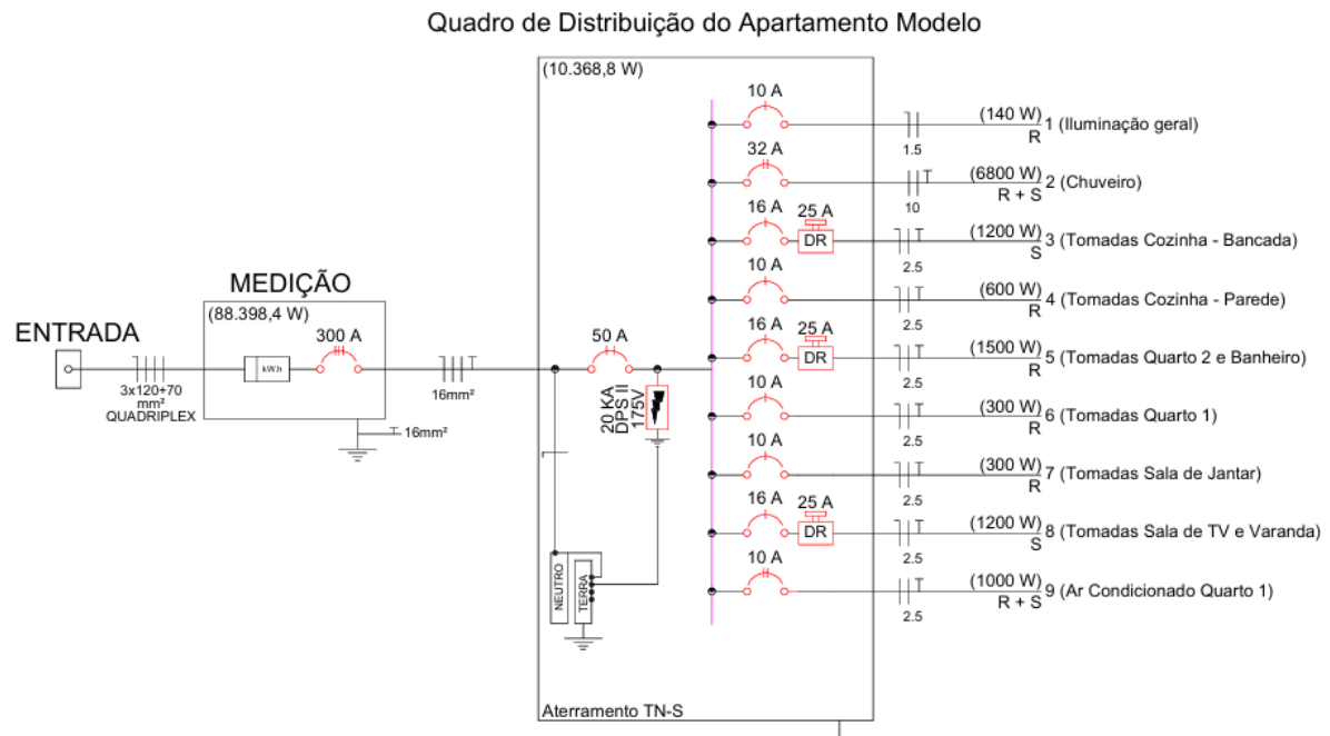
Figura 7 - Diagrama unifilar do apartamento modelo
